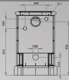
Teplovzdušný
